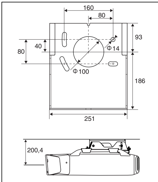
Gabarit de plafond (unités : mm)
