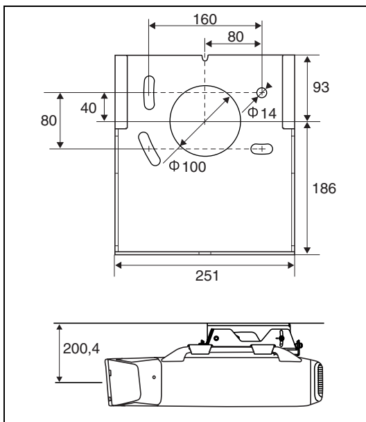
Plantilla para el techo (unidad: mm)
