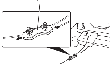
Presilla para cable
