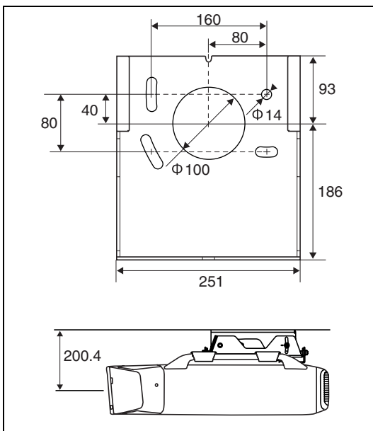
天井設置面寸法図（単位：mm）
