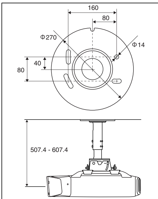
天花板樣板（單位：mm）
