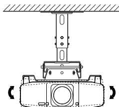
水平轉動調整
