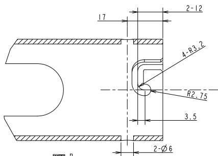
詳細図 B スケール 1.000
